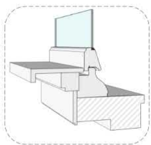
ondersnede N Kozijn C1
